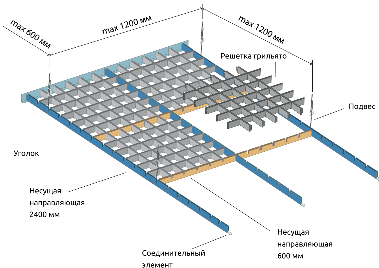
Высота профиля 40/50 мм Ширина профиля 10 мм
