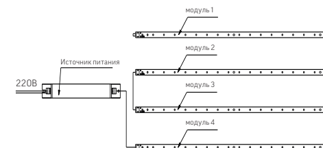
Рисунок 1. Подключение светильника к сети электропитания.
